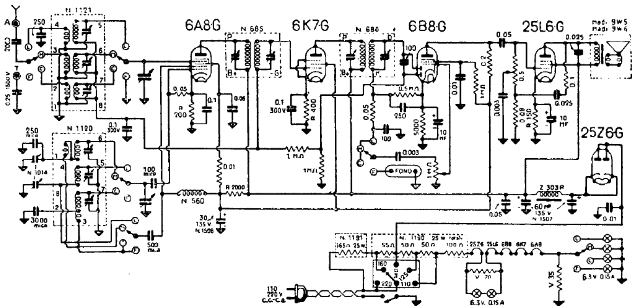
S. A. GELOSO. — Mod. G. 56. — Alimentazione: continua-alternata. — Media frequenza: 467 kHz. — Produzione 1935-1936.
